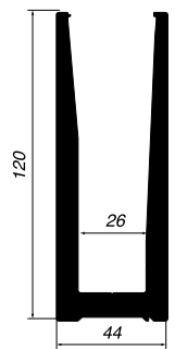
48.5028 Anclaje a forjado
